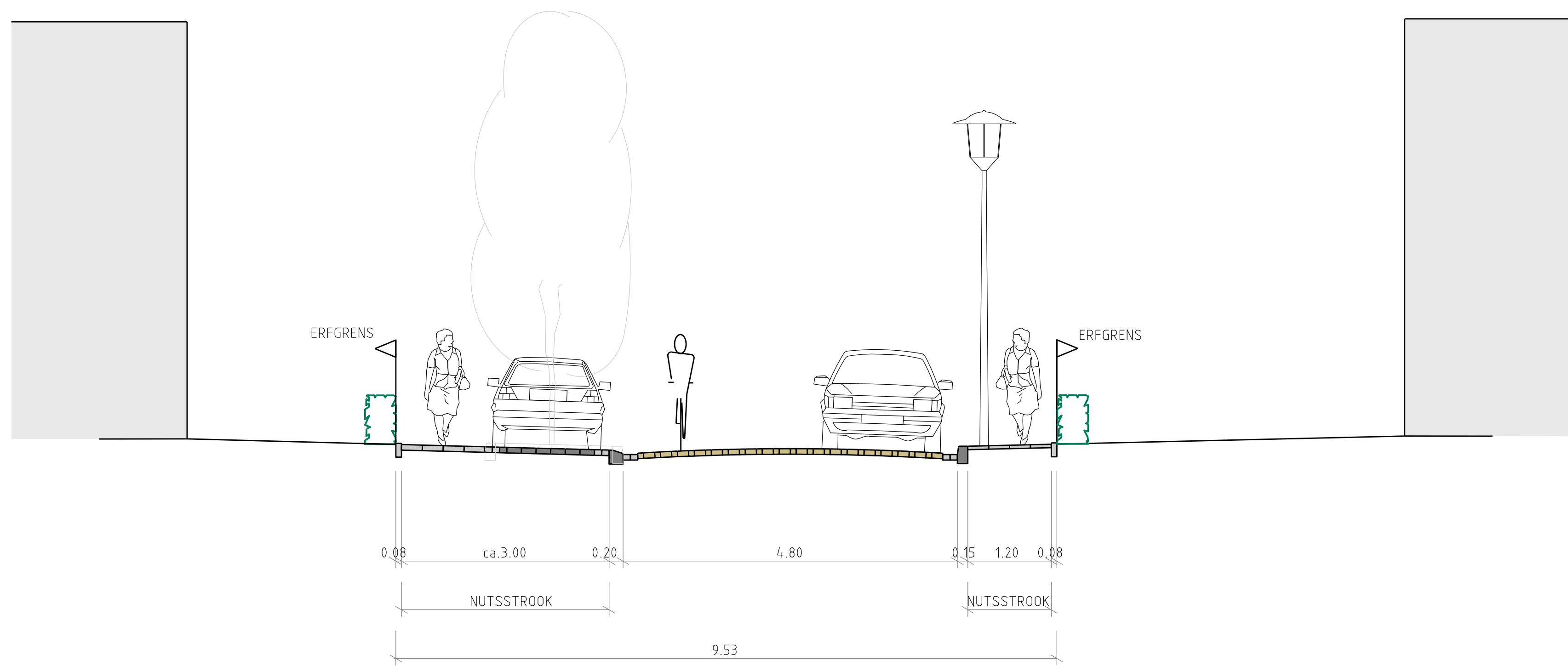
PRINCIPEPROFIEL VLASAKKERS
